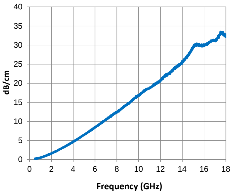
Attenuation
